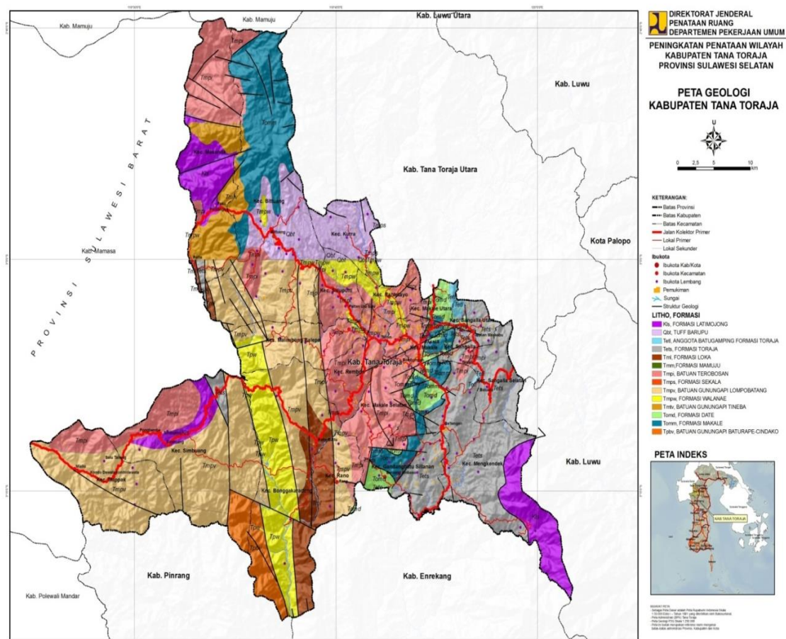
Gambar 2.5 Peta Geologi Kabupaten Tana Toraja
